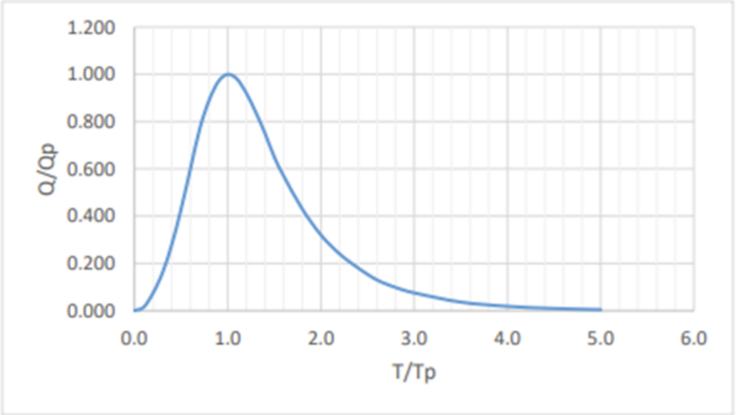
Gráfica HDR-L-1. Hidrograma unitario adimensional SCS
