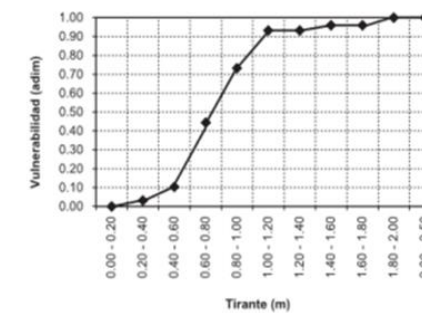
Función de vulnerabilidad para vivienda tipo III
