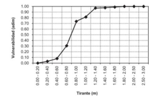
Función de vulnerabilidad para vivienda tipo V
