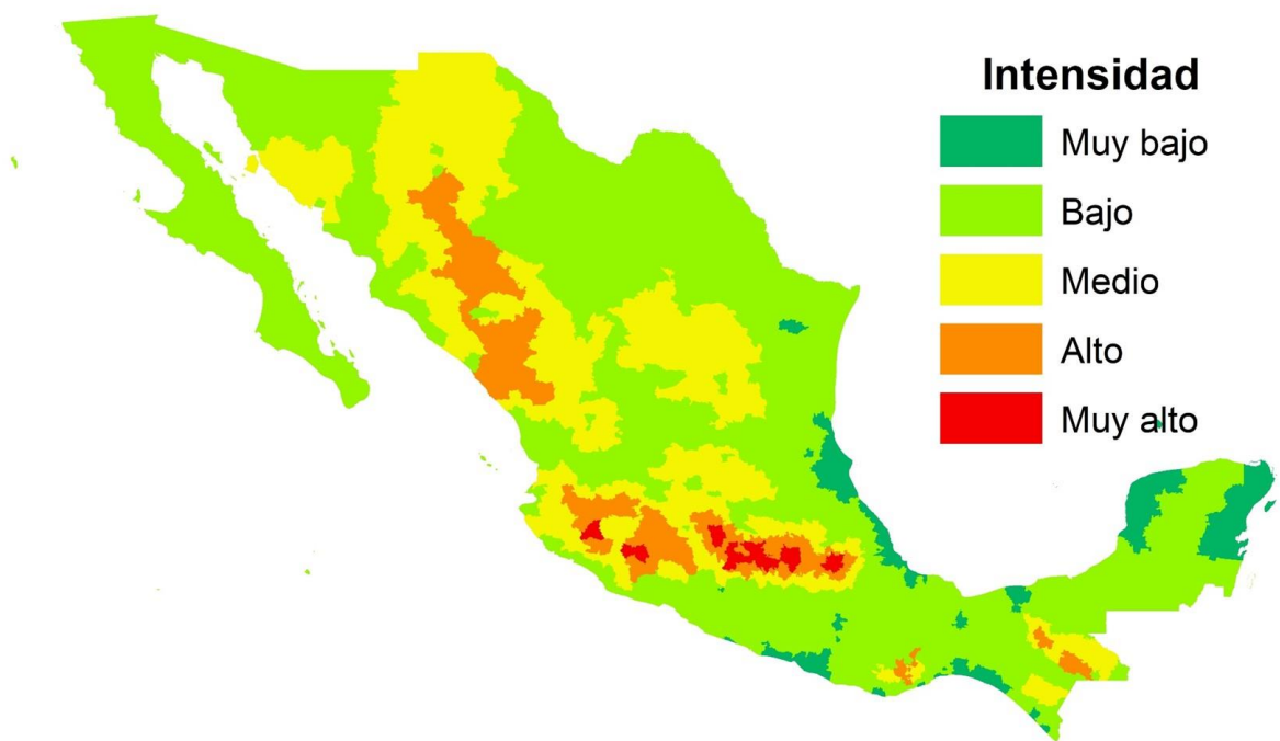
Imagen HDR-B-2. Intensidad de las granizadas en México
