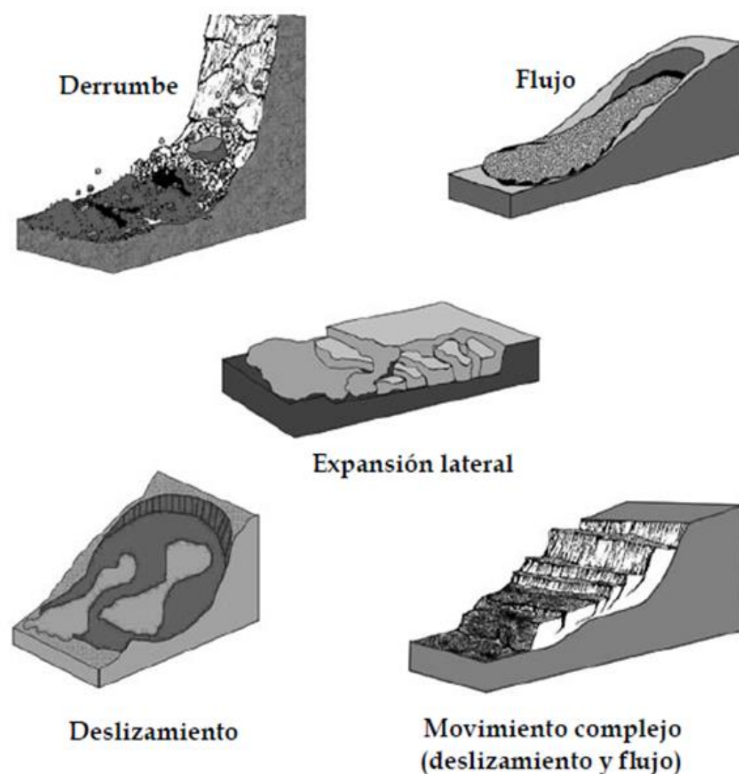
Imagen GEO-A-1. Tipos de procesos de remoción en masa.
