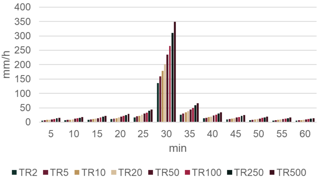
Gráfica HDR-E-1. Histograma por cada periodo de retorno, precipitación acumulada por instante de tiempo.
