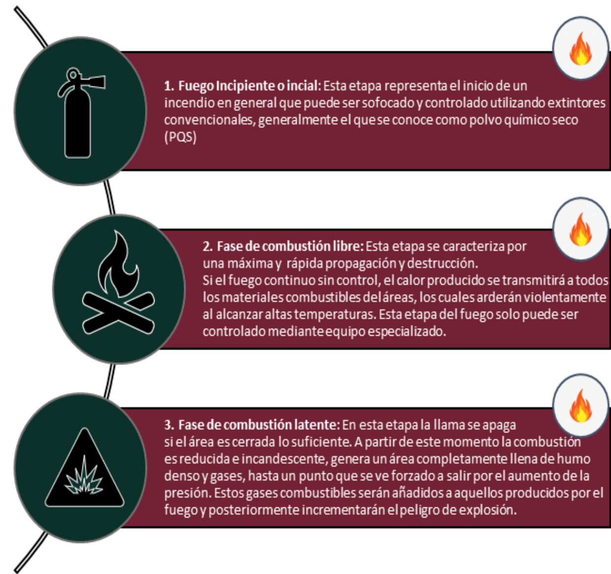
Diagrama QTC – D – 1. Fases de un incendio
