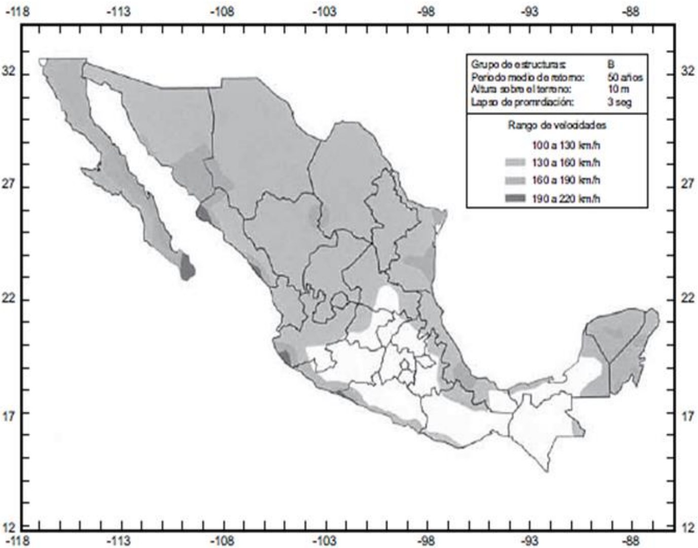
Imagen HDR-A. Zonificación de velocidades máximas de viento en la República Mexicana.
