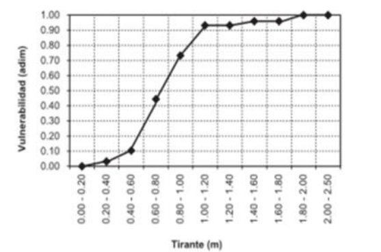
Función de vulnerabilidad para vivienda tipo III
