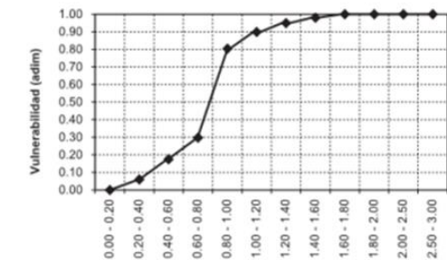
Función de vulnerabilidad para vivienda tipo IV
