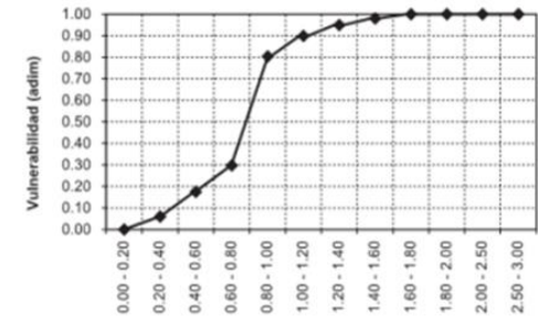
Función de vulnerabilidad para vivienda tipo II
