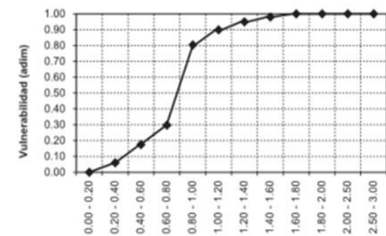
Función de vulnerabilidad para vivienda tipo II
