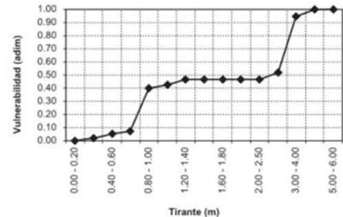
Función de vulnerabilidad para vivienda tipo IV
