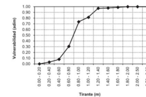
Función de vulnerabilidad para vivienda tipo V
