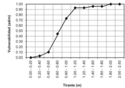
Función de vulnerabilidad para vivienda tipo III
