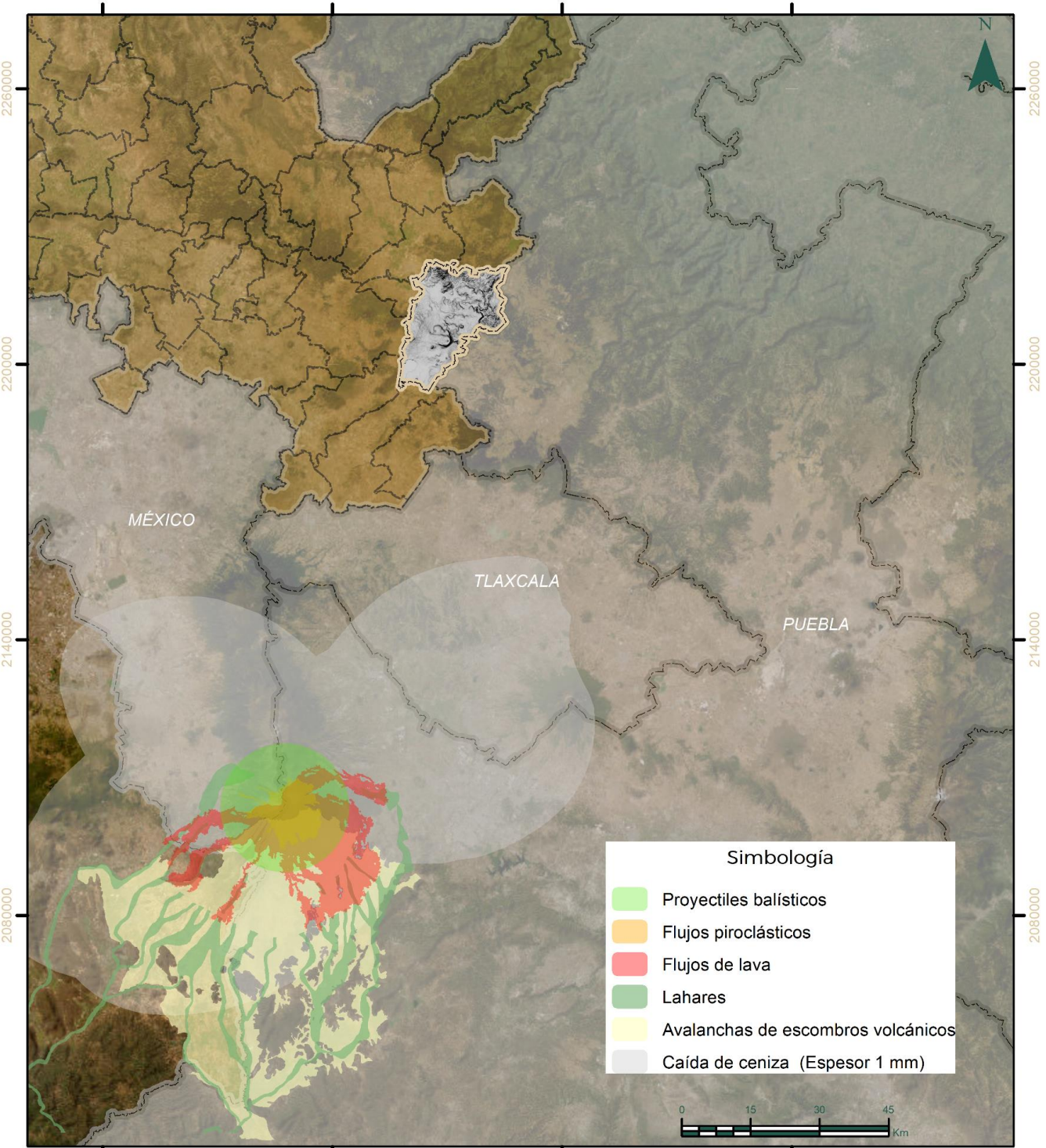
Imagen GEO-D-4. Mapa de peligros volcánicos del Popocatepetl y su influencia en Cuauteppec
