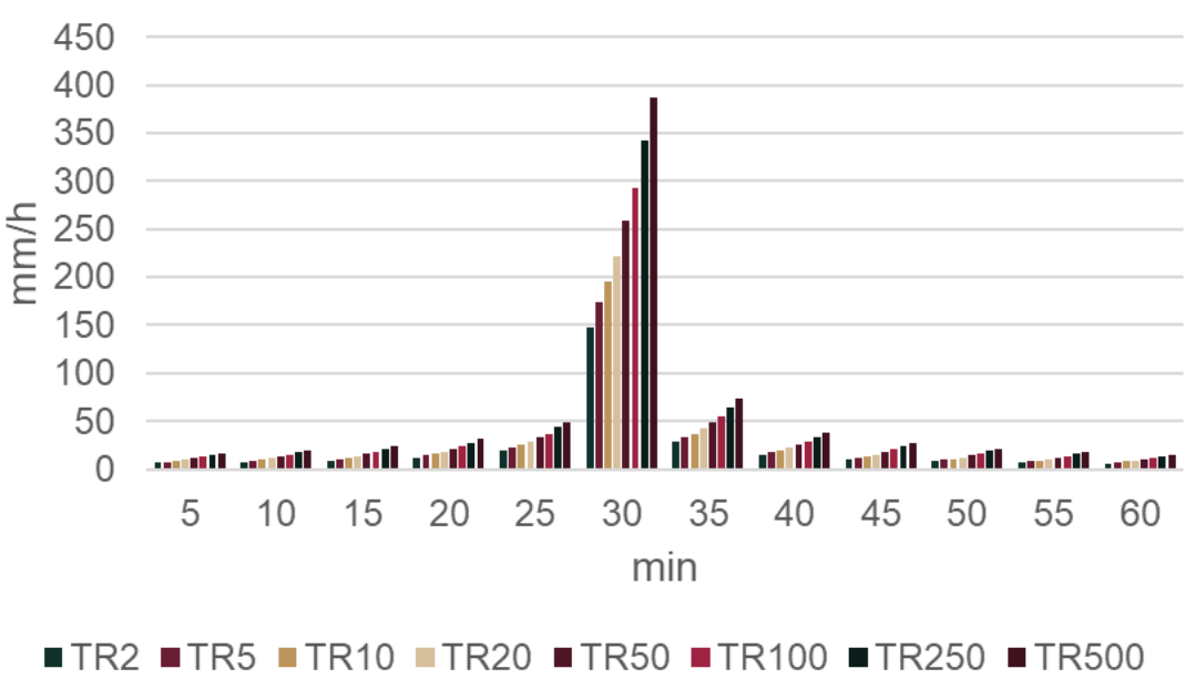
Gráfica HDR-B-1. Histograma por cada periodo de retorno, precipitación acumulada por instante de tiempo.
