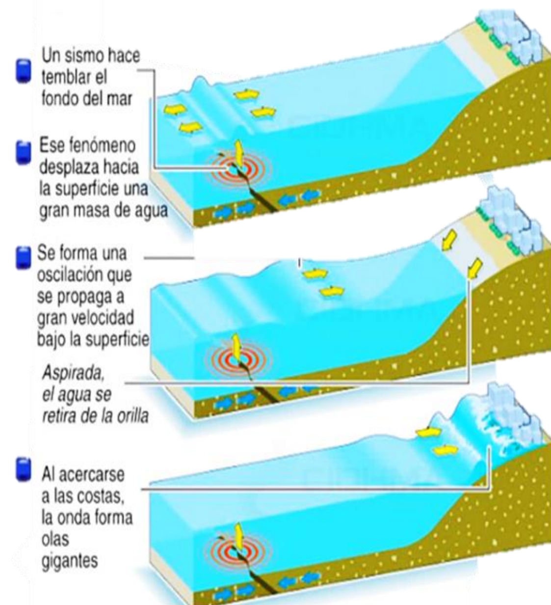
Imagen GEO-C. Formación de un Tsunami.
