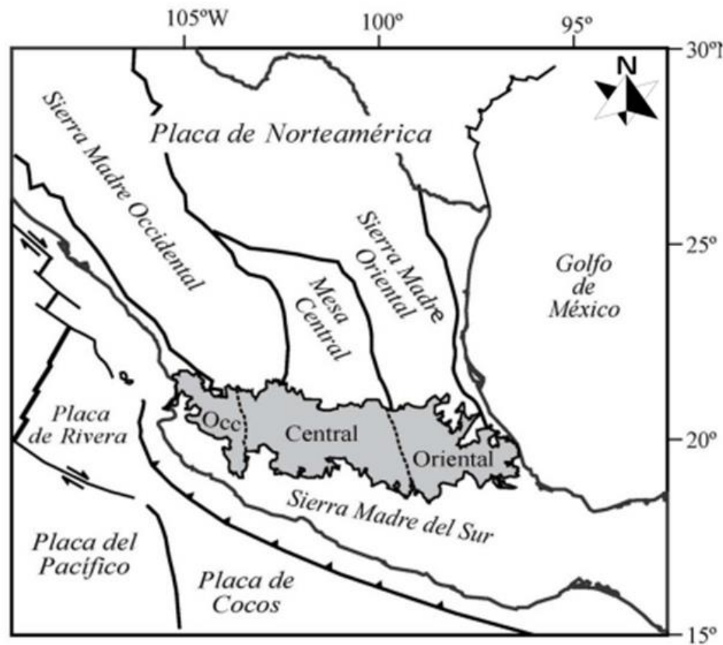
Imagen GEO-B-4. Descripción tectónica del centro
