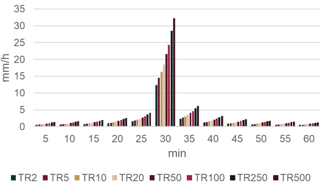
Gráfica HDR-B-2. Histograma por cada periodo de retorno, precipitación acumulada por instante de tiempo.
