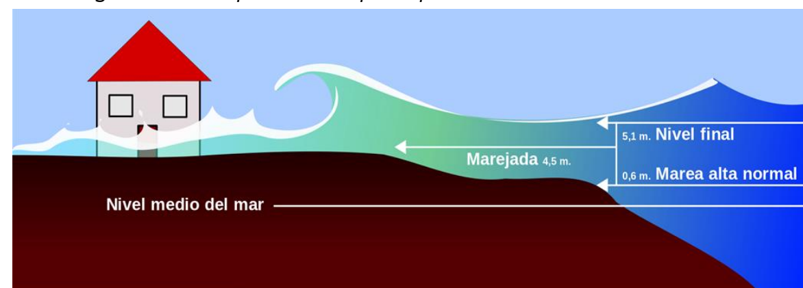
Imagen HDR-D. Esquema del impacto por fenómeno de marea de tormenta.
