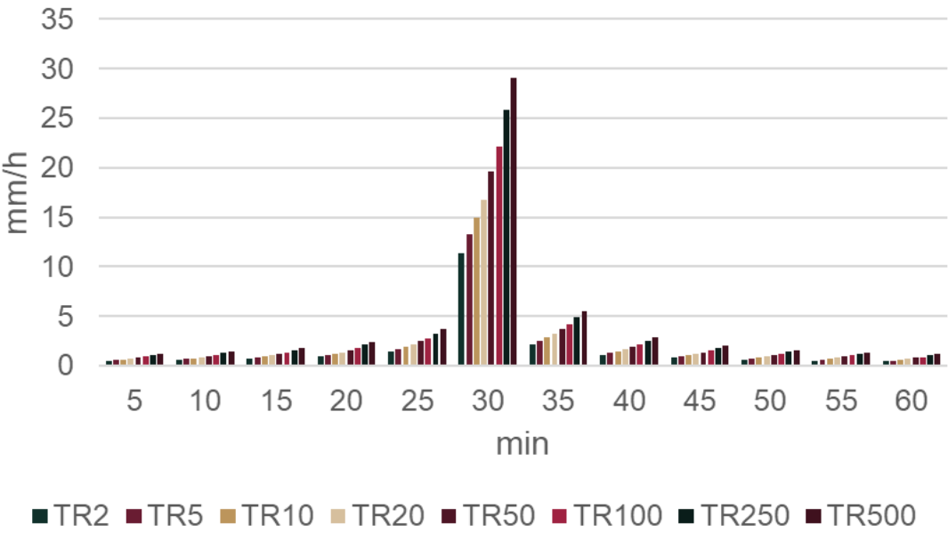
Gráfica HDR-E-20. Histograma por cada periodo de retorno, precipitación acumulada por instante de tiempo.
