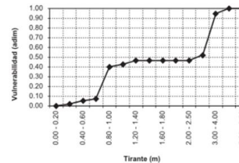
Función de vulnerabilidad para vivienda tipo V
